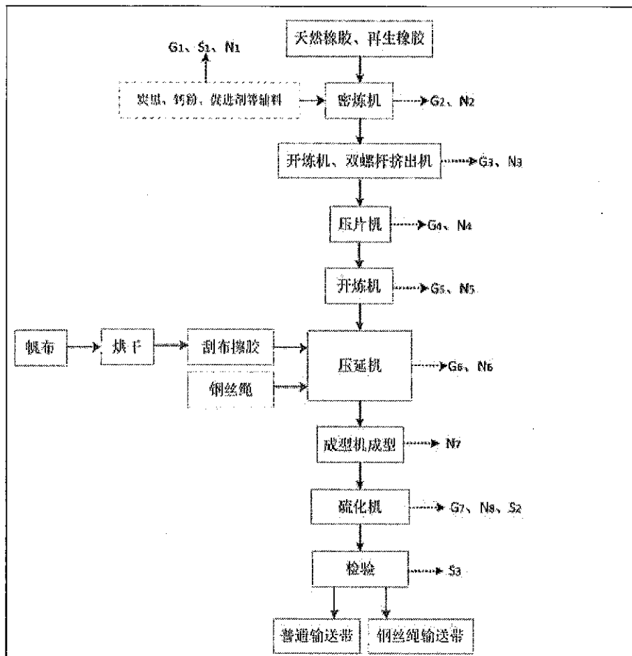
图3-2 受核查方主要生产流程图
